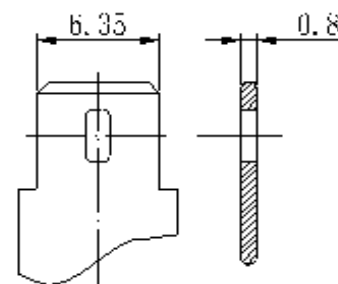
Клеммы
