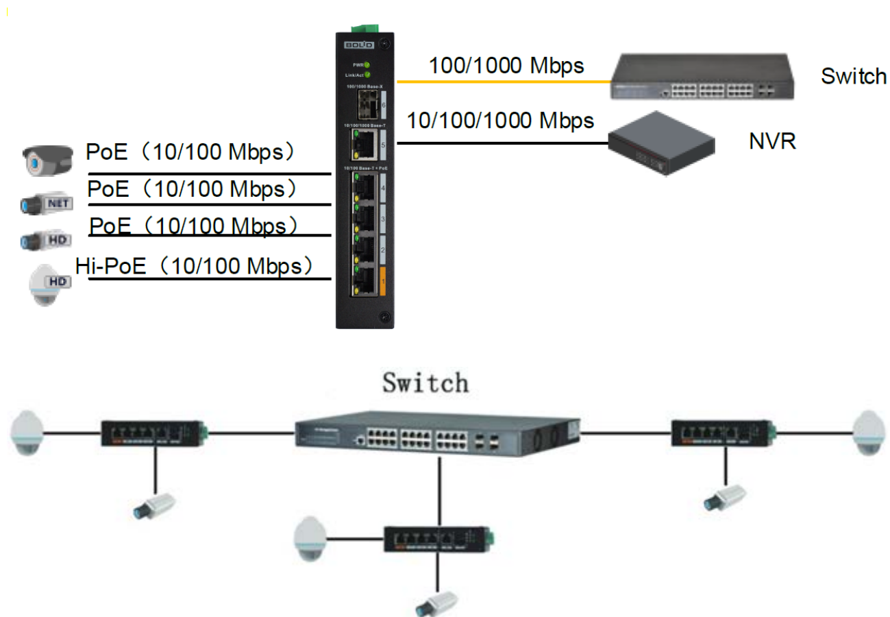
Рисунок 1.1 – Сетевое соединение
