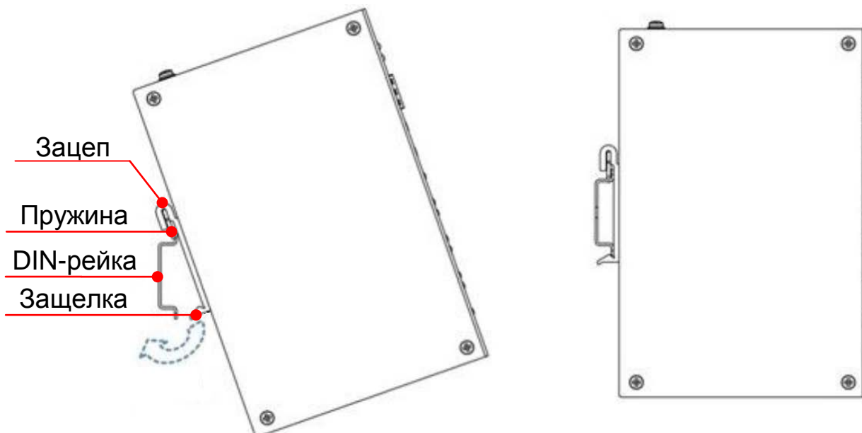
Рисунок 5.3 – Инсталляция
