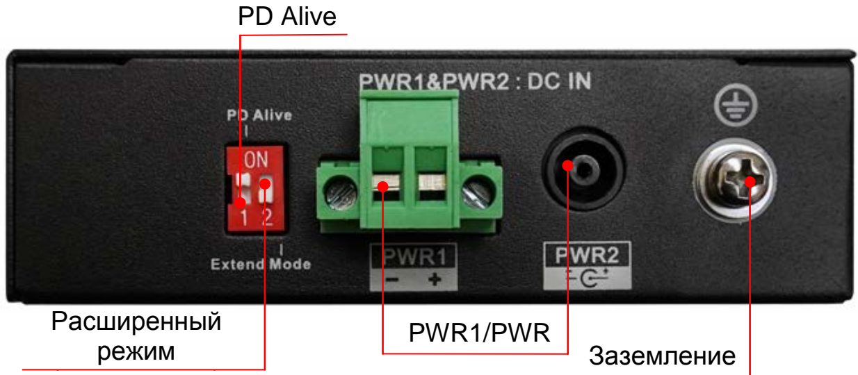
Рисунок 5.1 – Верхняя панель
