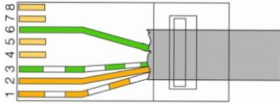
Схема обжима при использовании 2-х парного кабеля по стандарту T-568B
