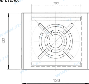
Рис.1 Габаритные размеры
