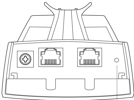
Кнопка RESET Нажмите и удерживайте в течение 8 секунд
