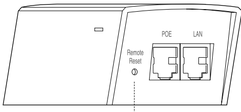
Кнопка Remote reset Нажмите и удерживайте 8 секунд
