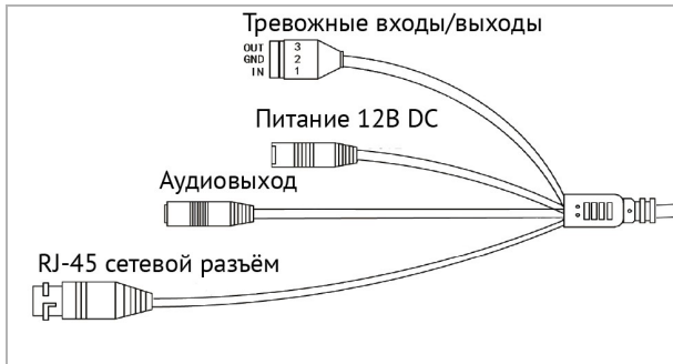
TR-D2221WDIR4W
