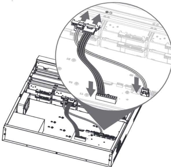
Рисунок 3.8 – Установка жесткого диска
