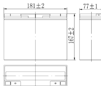
Габариты
